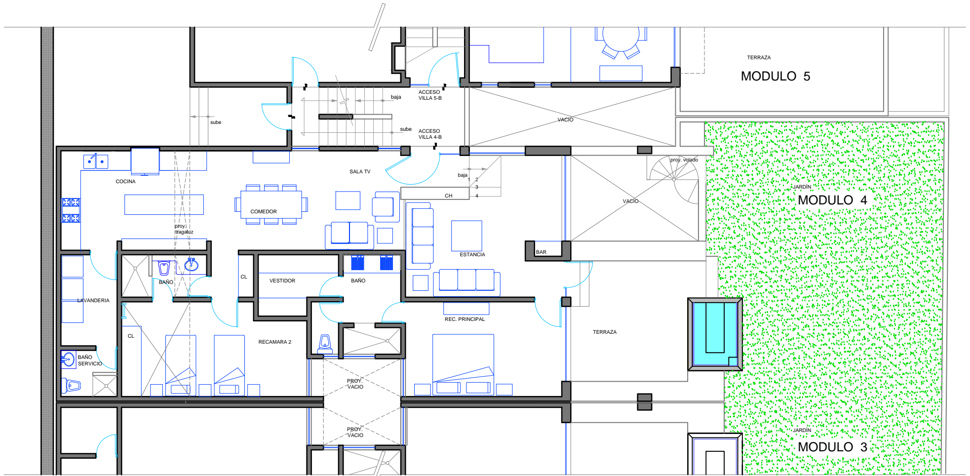
NIVEL -1 PLANTA UNICA CASA 4-B
